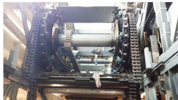
Demontierte Antriebseinheit
